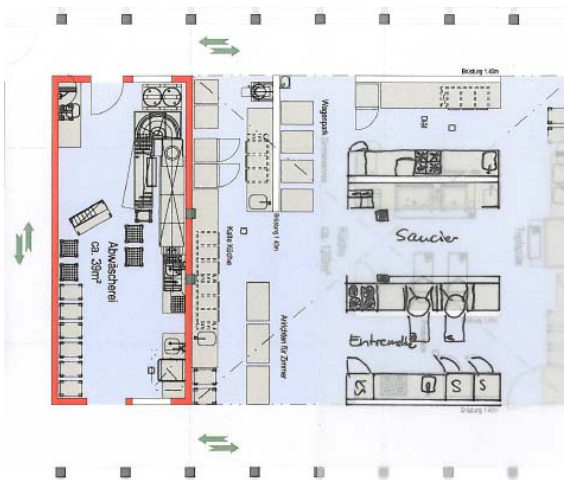
Skizze Vorprojekt Abwäscheri und Küche (Ausschnitt)
